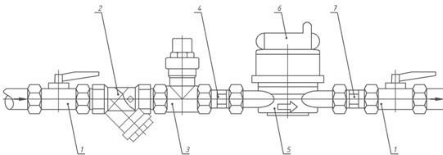
Типовая схема монтажа индивидуального узла учета воды потребителя
